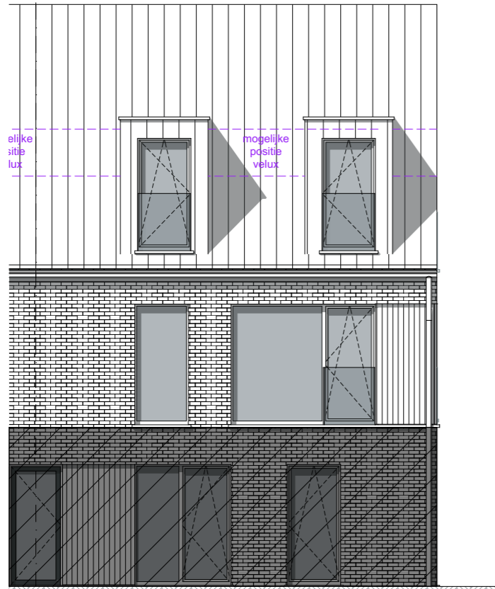
VOORGEVEL
