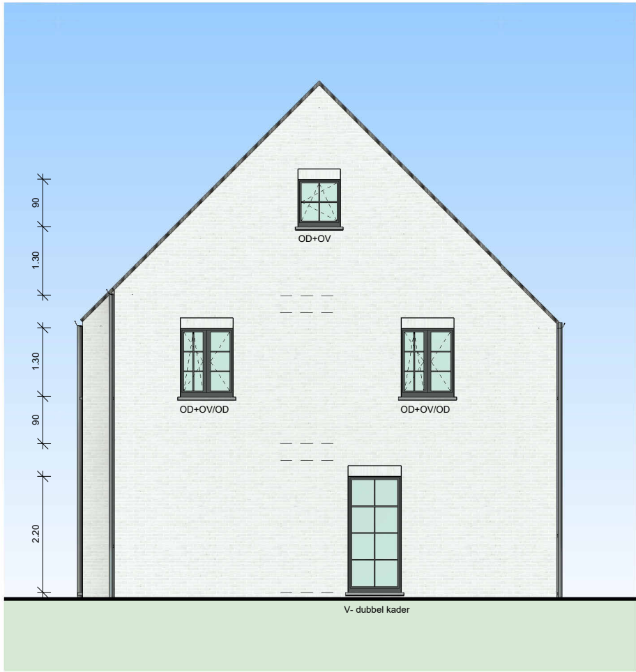
Voorgevel
