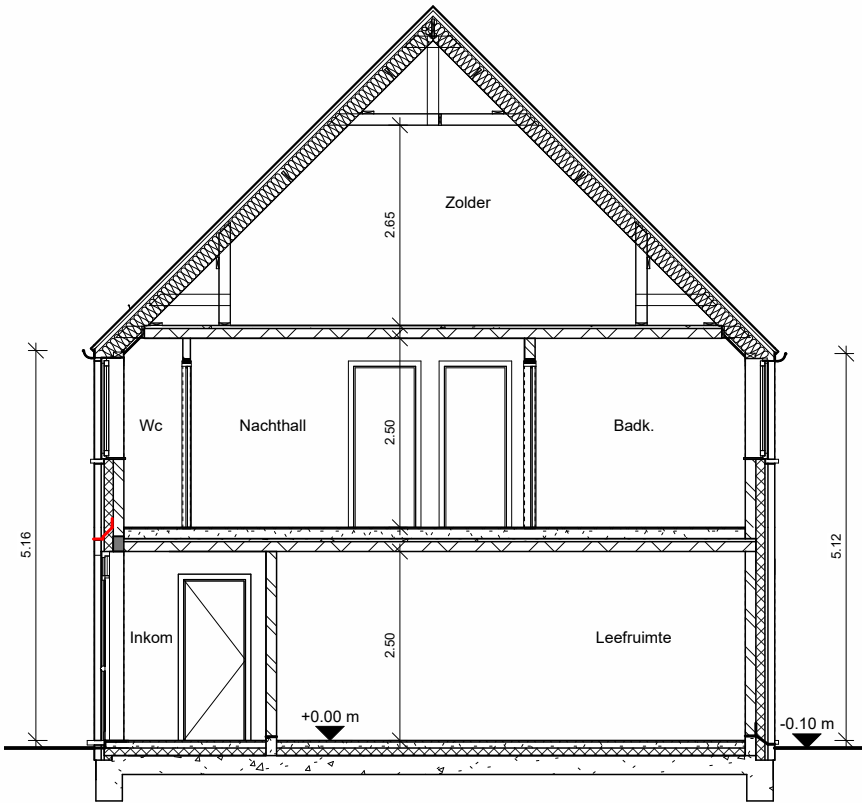
Doorsnede
