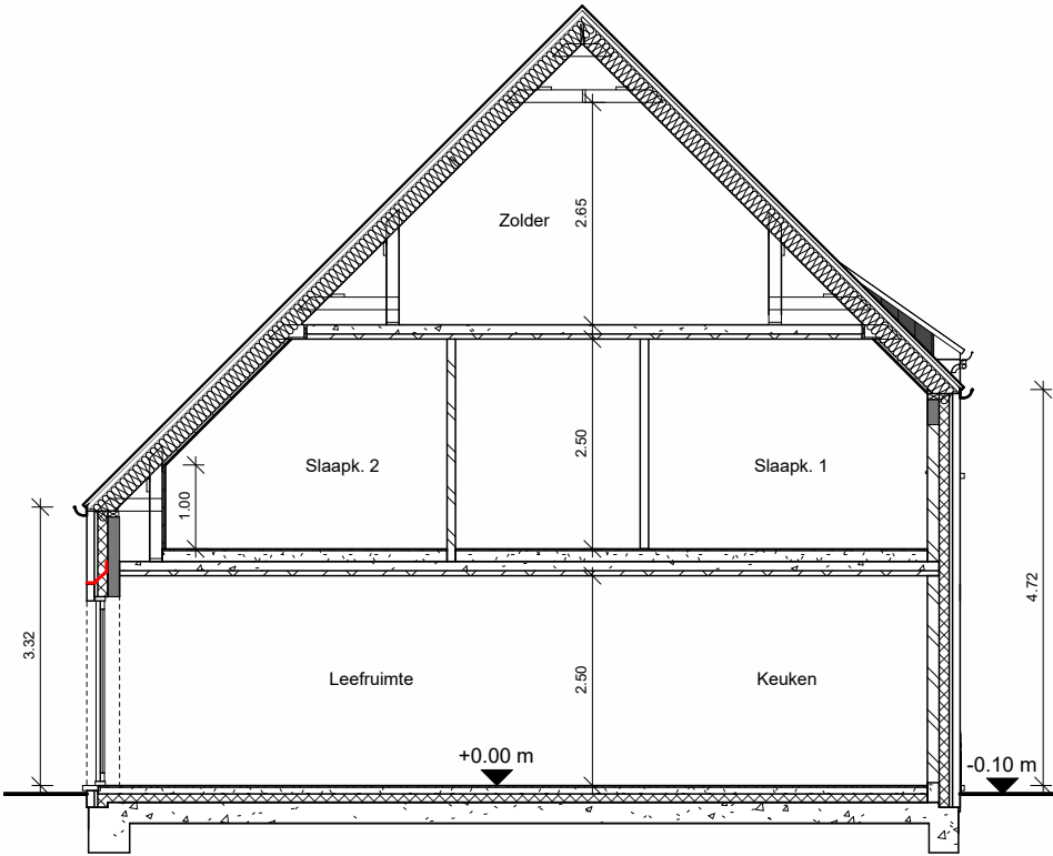
Doorsnede 2
