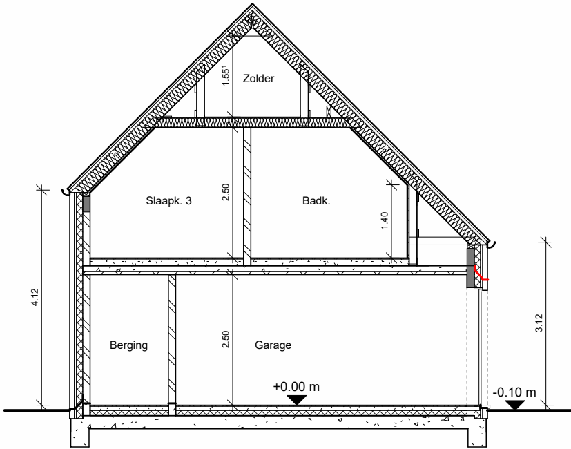
Doorsnede 1
