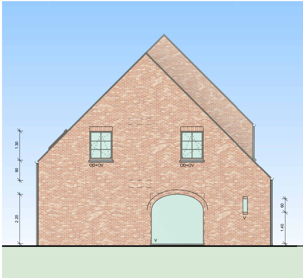
Zijgevel
