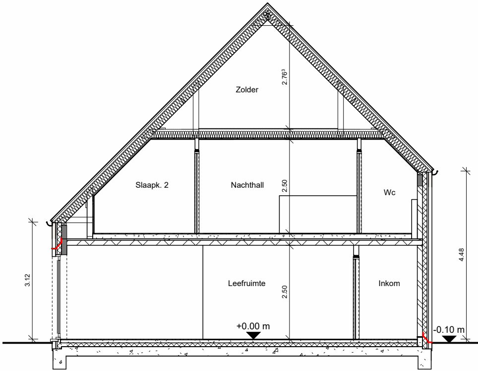
Doorsnede 2
