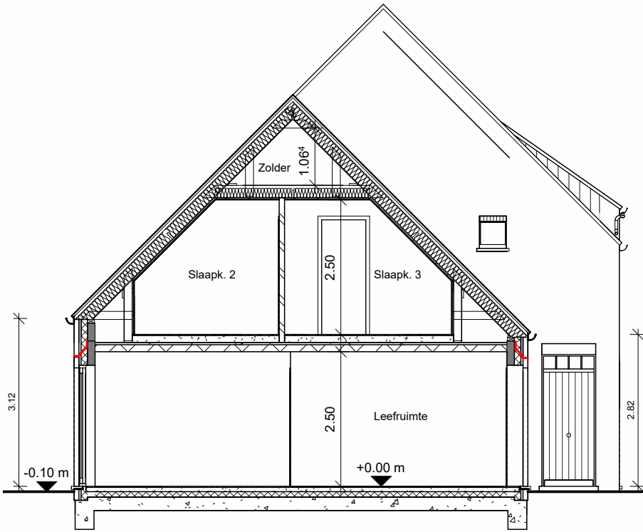
Doorsnede 1
